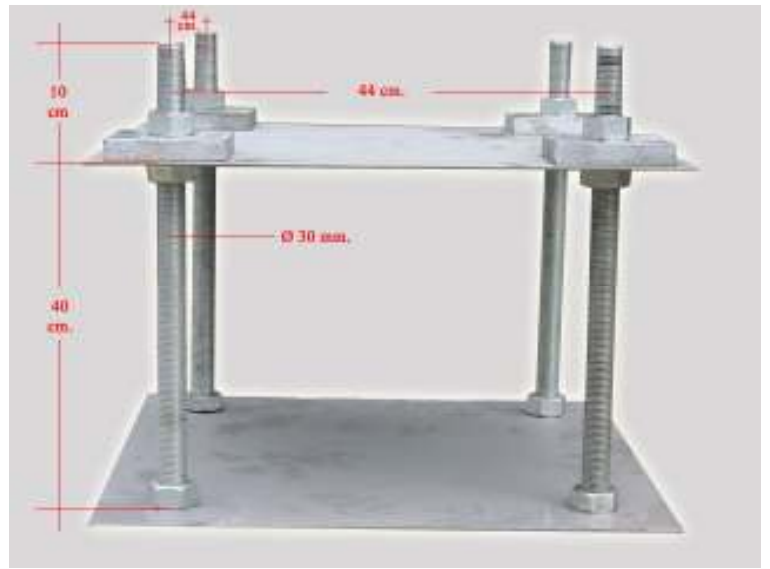
Resim 01 – Beton Şablonu
